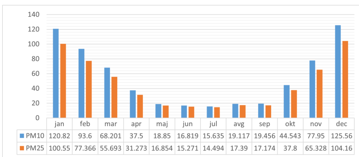
Grafikon 1 Prosečne koncentracije PM 10 i PM 2.5 po mesecima u periodu od 2021. do 2023. godine.
